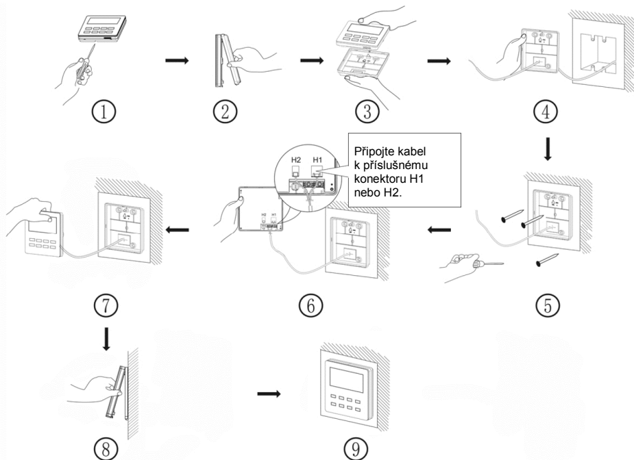
Obr. 23: Postup instalace kabelového ovladače
