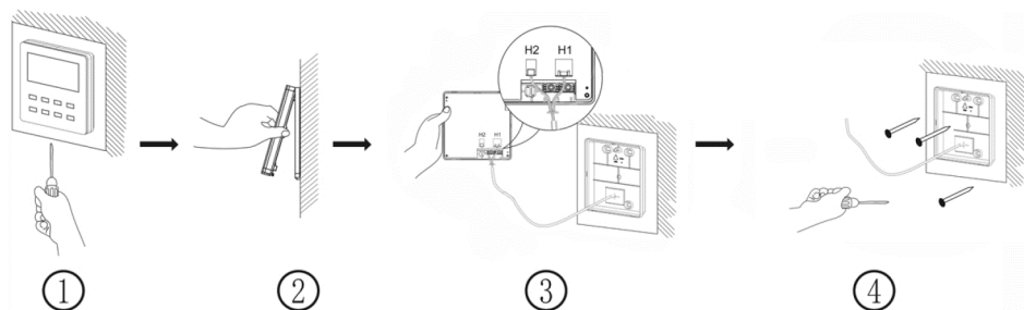
Obr. 24: Postup demontáže kabelového ovladače
