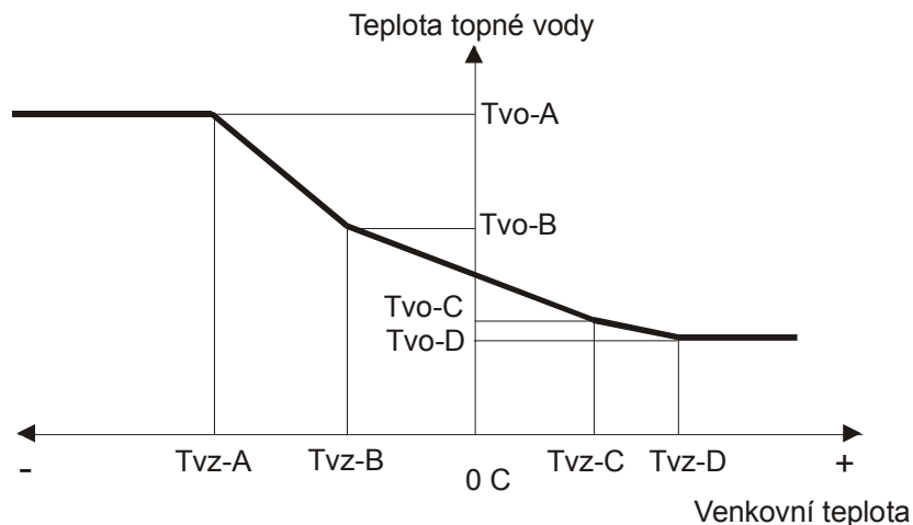
Obr. 4. Ekvitermní křivka
